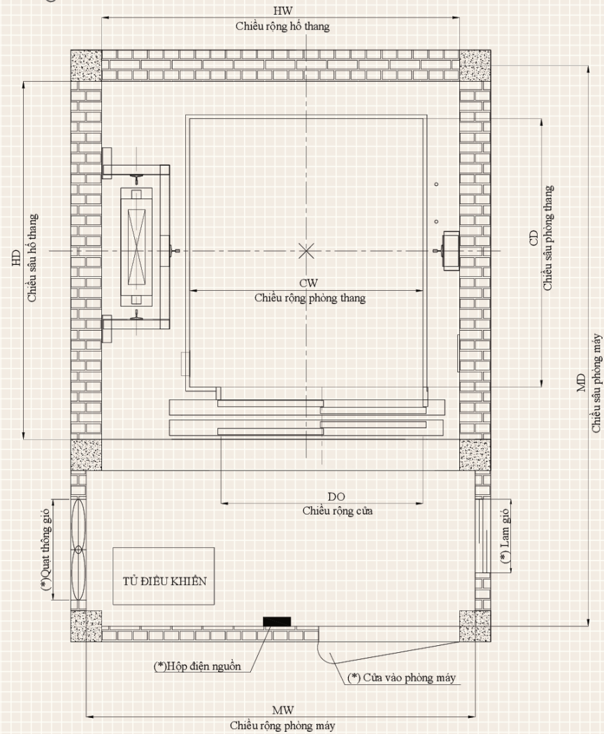
2SO Type Section / Mặt Cắt Ngang Hố Thang Cửa 2SO
